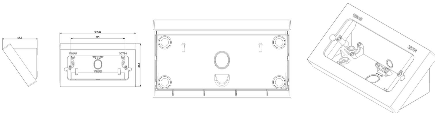
Vista ingombri
