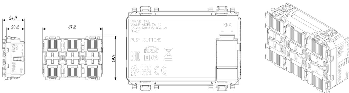
Vista ingombri
