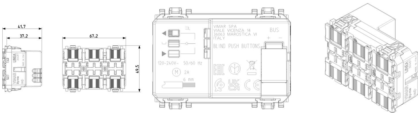
Vista ingombri
