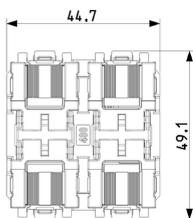
Vista ingombri
