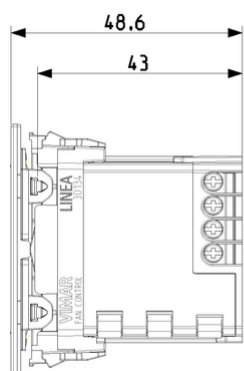
Vista ingombri
