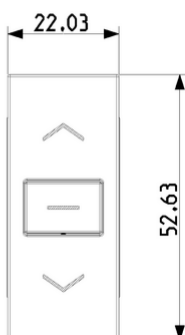
Vista ingombri
