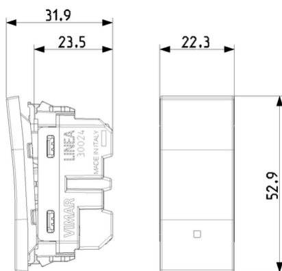
Vista ingombri
