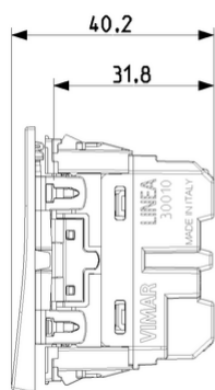
Vista ingombri
