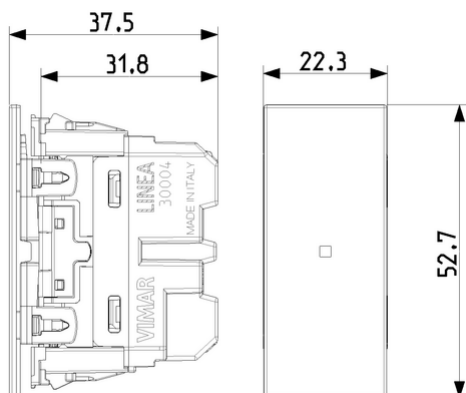
Vista ingombri
