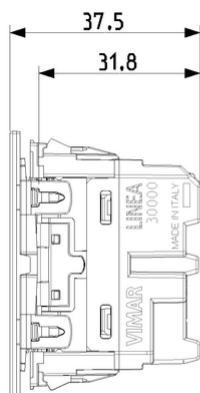
Vista ingombri
