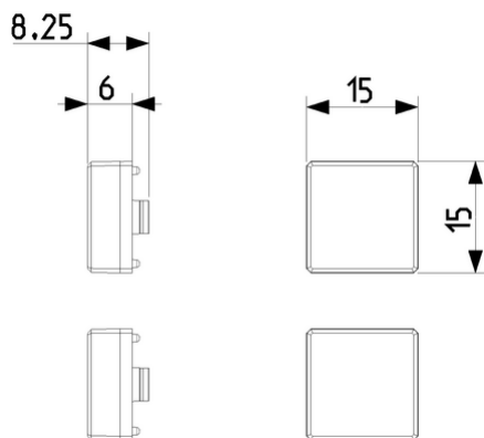
Vista ingombri
