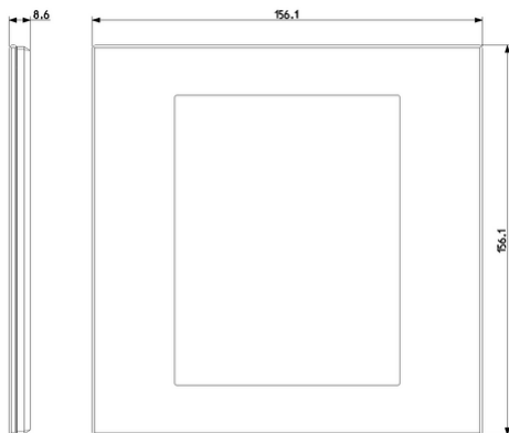
Vista ingombri
