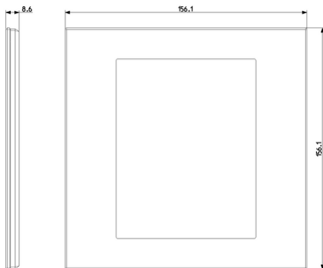
Vista ingombri
