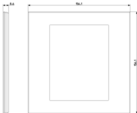
Vista ingombri
