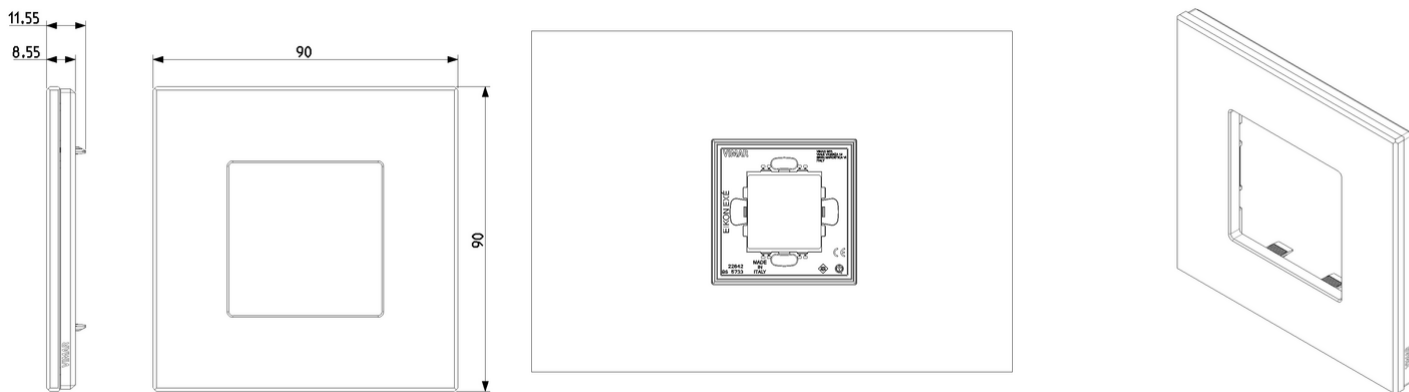
Vista ingombri
