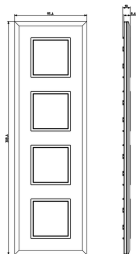
Vista ingombri
