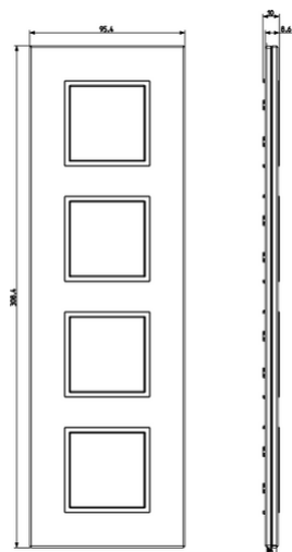
Vista ingombri
