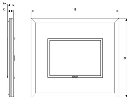
Vista ingombri
