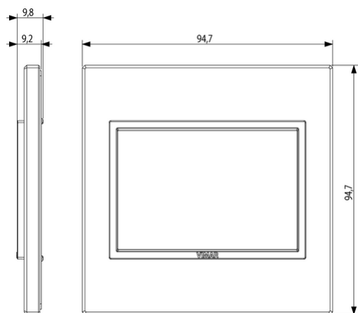
Vista ingombri
