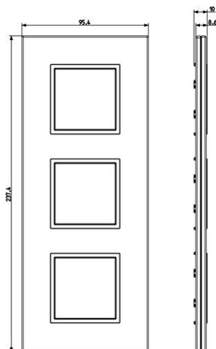
Vista ingombri
