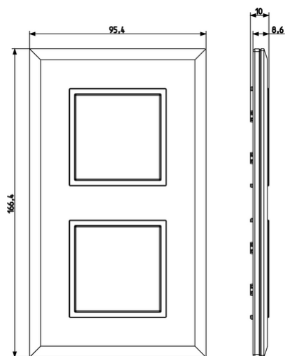
Vista ingombri
