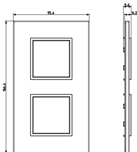
Vista ingombri
