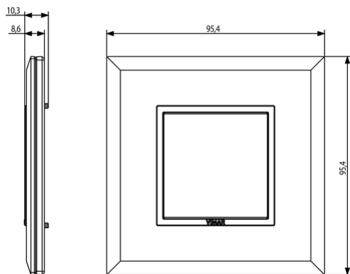
Vista ingombri
