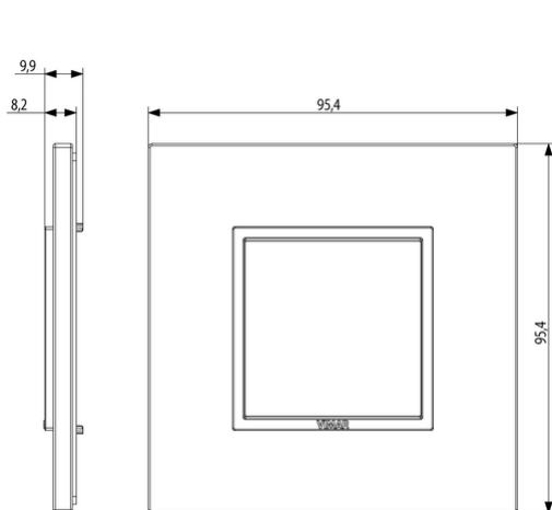
Vista ingombri
