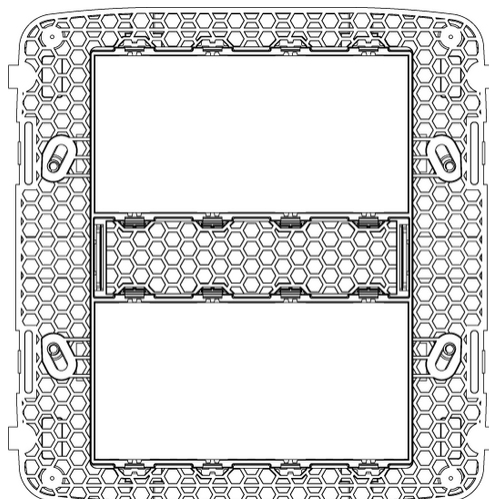
Vista posteriore
