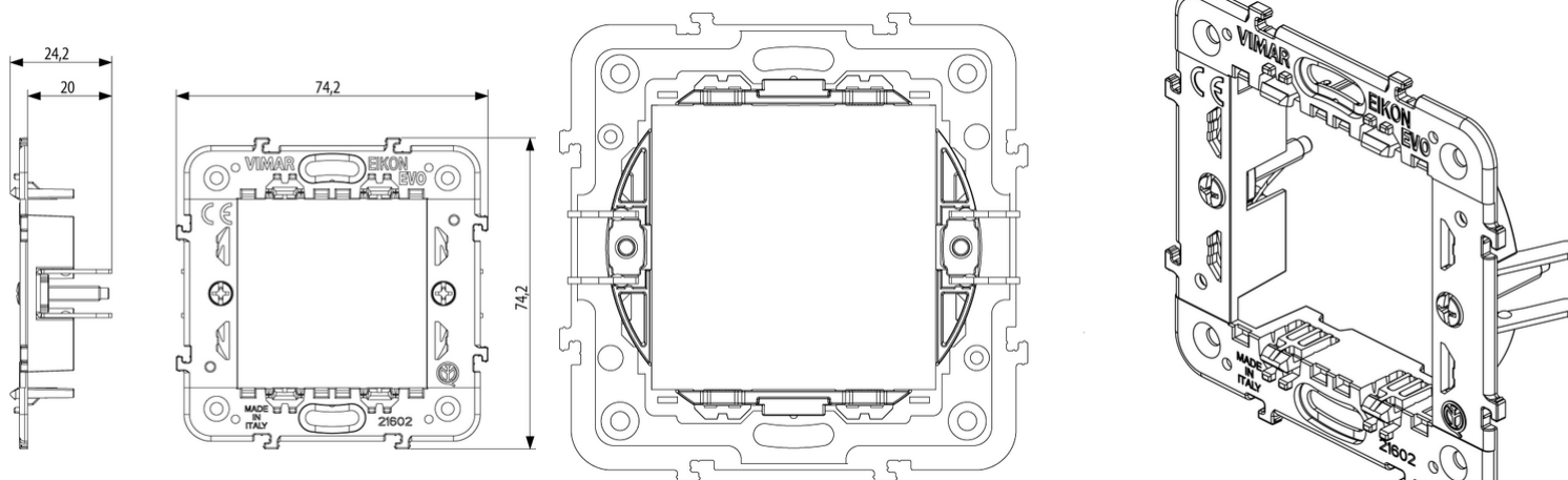
Vista ingombri
