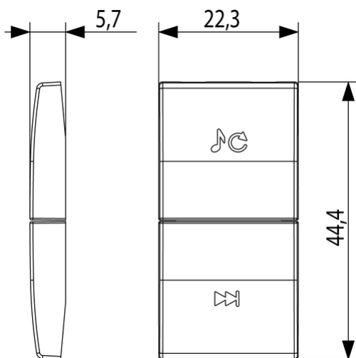
Vista ingombri
