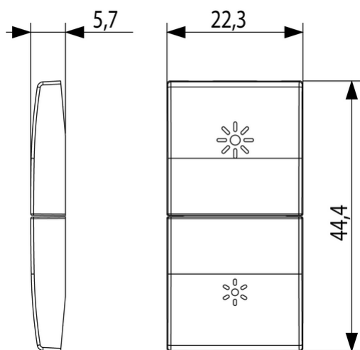
Vista ingombri
