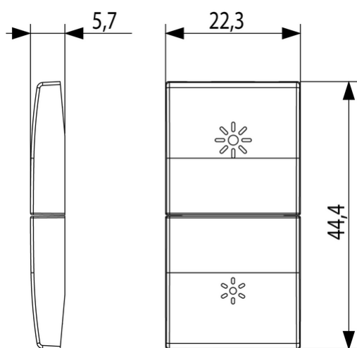
Vista ingombri
