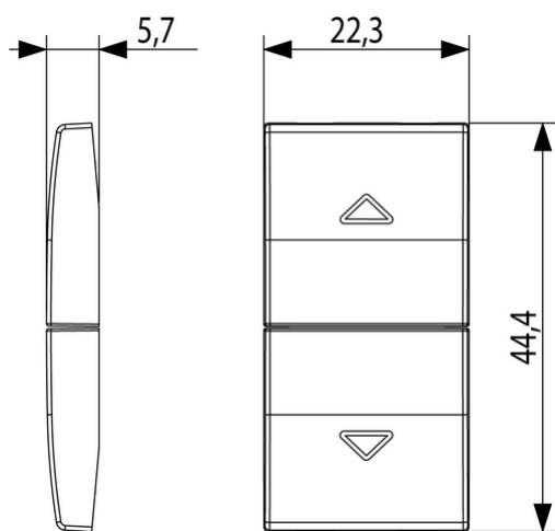
Vista ingombri
