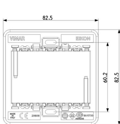
Vista ingombri
