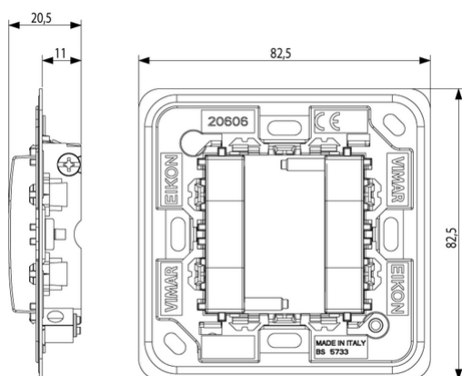
Vista ingombri
