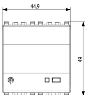
Vista ingombri
