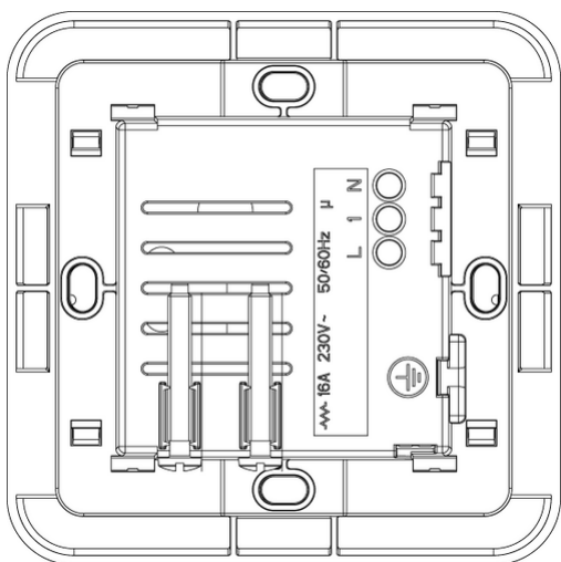
Vista posteriore
