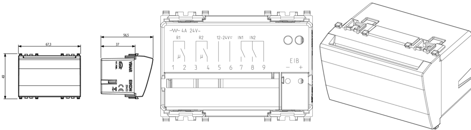
Vista ingombri
