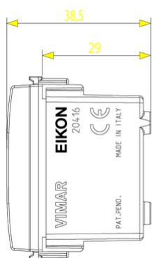
Vista ingombri
