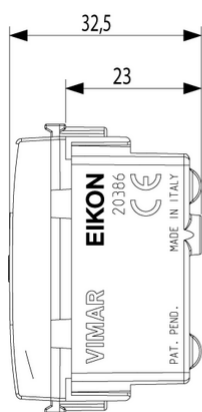
Vista ingombri
