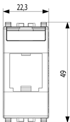
Vista ingombri
