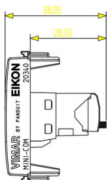
Vista ingombri
