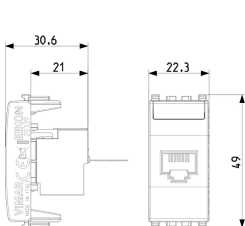
Vista ingombri
