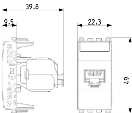
Vista ingombri
