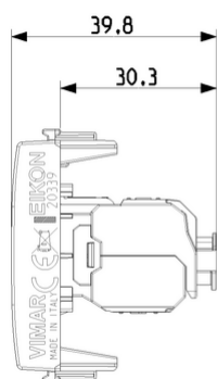
Vista ingombri
