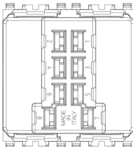
Vista posteriore
