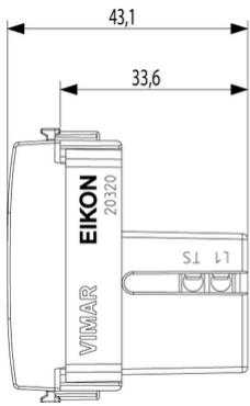
Vista ingombri
