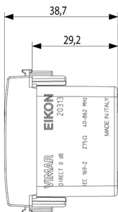
Vista ingombri
