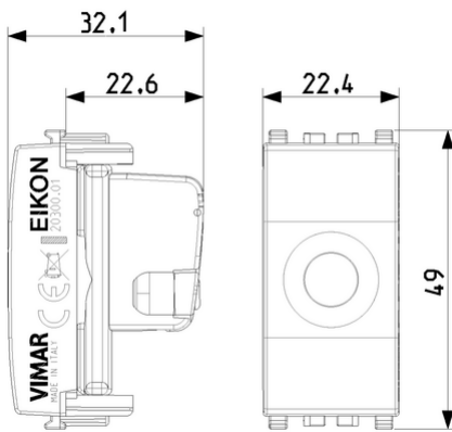
Vista ingombri
