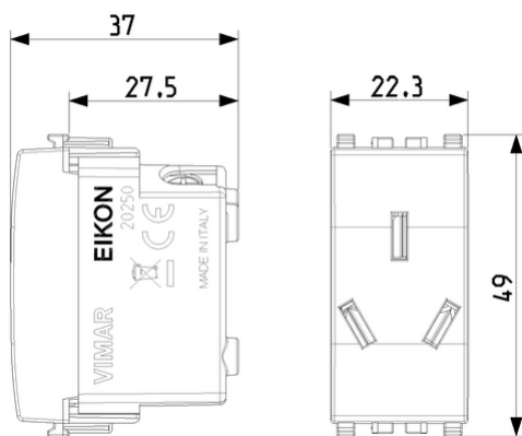
Vista ingombri
