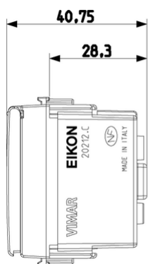
Vista ingombri
