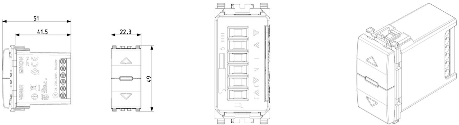
Vista ingombri
