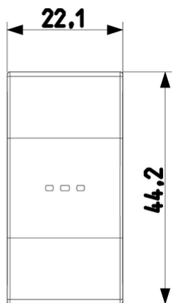
Vista ingombri
